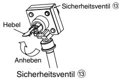
Sicherheitsventil 13
