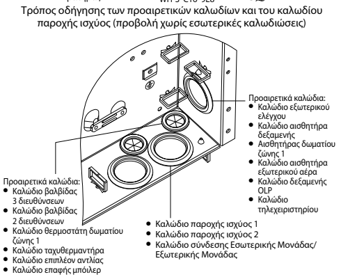
Τρόπος οδήγησης των προαιρετικών καλωδίων και του καλωδίου παροχής ισχύος (προβολή χωρίς εσωτερικές καλωδιώσεις)
