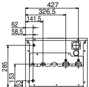
VISTA INFERIOR
