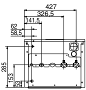
ANSICHT VON UNTEN
